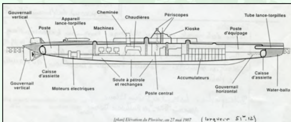
Schéma en coupe du sous marin Le Pluviôse
