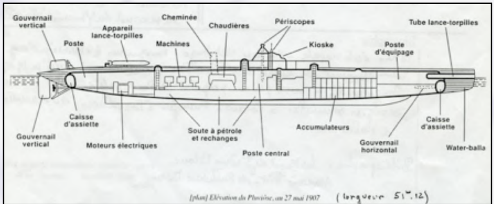
Schéma en coupe du sous marin Le Pluviôse
